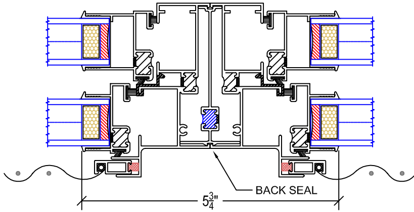
DH SHOWN w/ INTERNAL MULLION
